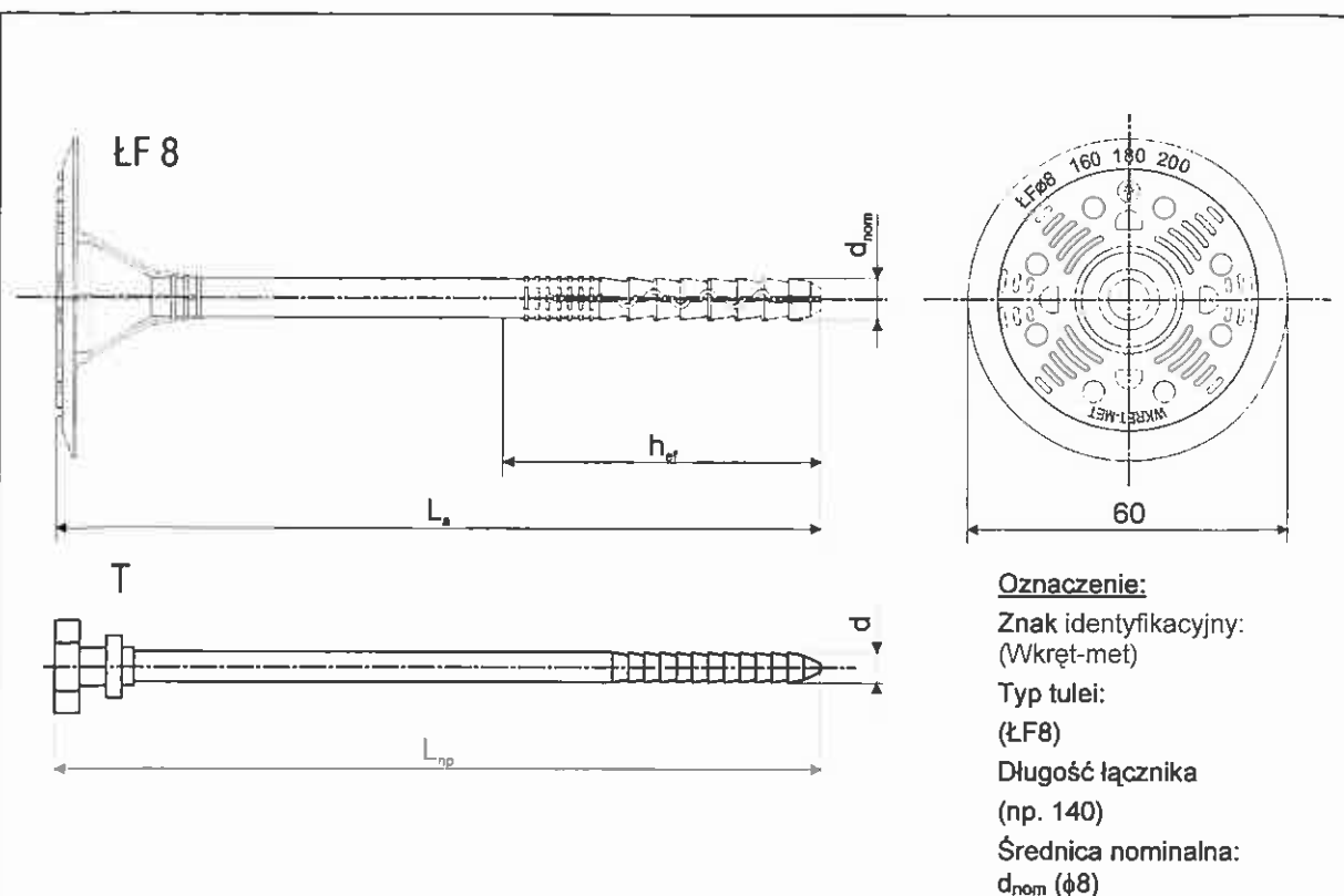
Tablica 1: Oznaczenia i wymiary [mm] łączników WKRET-MET-ŁFN \phi 8
