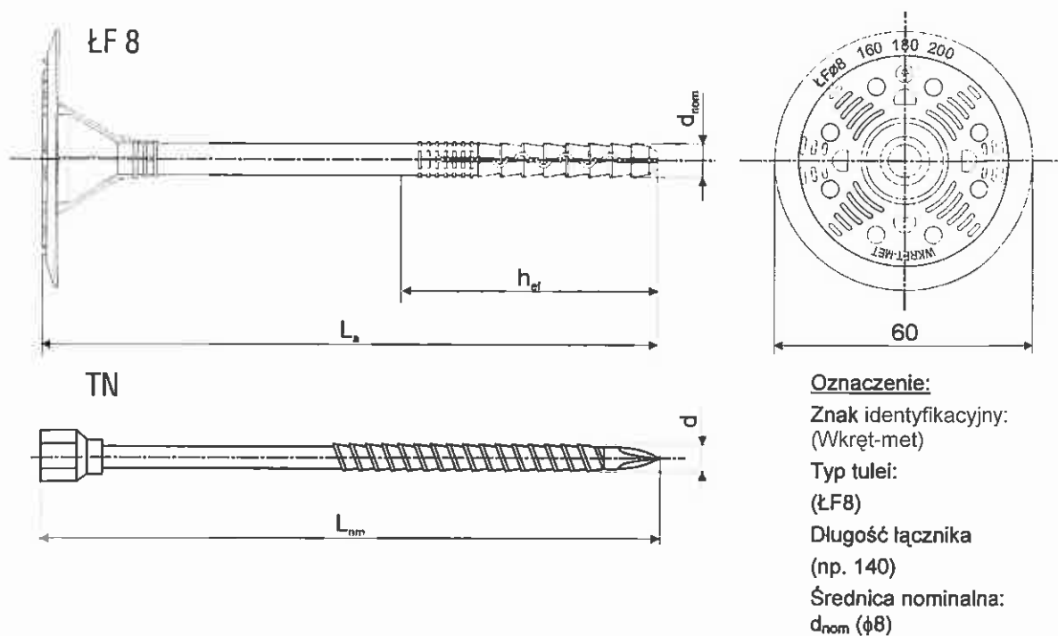
Tablica 2: Oznaczenia i wymiary [mm] łączników WKRET-MET-ŁFM \phi 8
